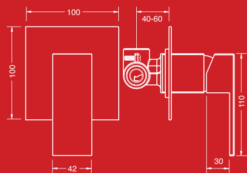
Wall Mixer ALS-SCW
